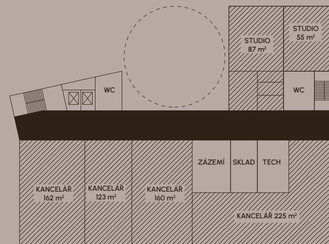
Půdorys kancelářského patra (3 NP, 4 NP)
