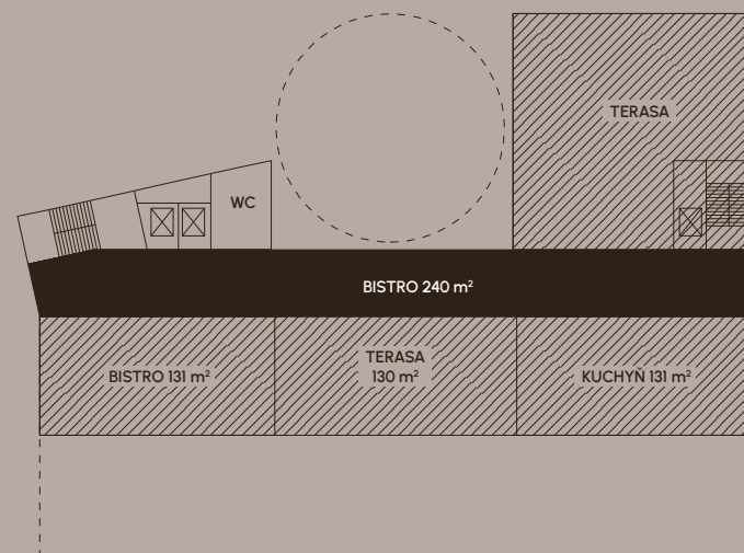
Půdorys posledního patra (6 NP)
