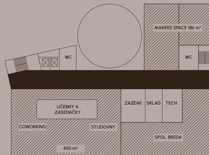
Půdorys druhého nadzemního patra v propojení kupoly (2 NP)
